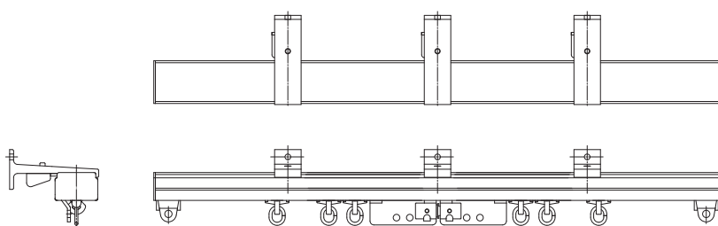
▲納まり図
