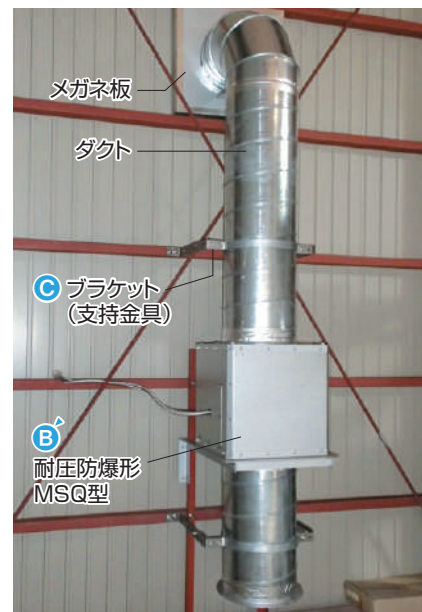
▲ 耐圧防爆形 MSQ型 (中間型) 〔屋内〕
