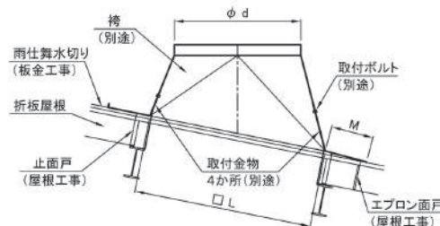
屋根設置 桁(オプション)納まり図
